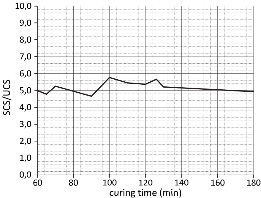
Fig. 9. Trend of SCS/UCS in function of curing time. Andamento del rapporto SCS/UCS in funzione del tempo di maturazione.
