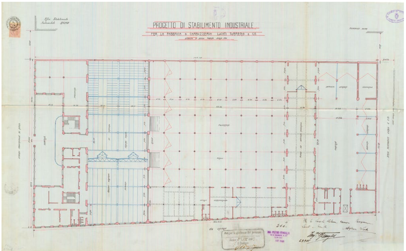
Figura 4. Pietro Fenoglio, planimetria dello stabilimento Locati-Torretta (ASCT, Progetti Edilizi, 1905, n. 366, tavola 2).
