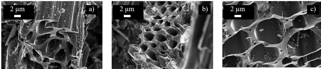
5 6 Fig. 3. FESEM images of a) MIS 650, b) MIS 700 and c) MIS 750 Biochars at 10kX magnifications.
