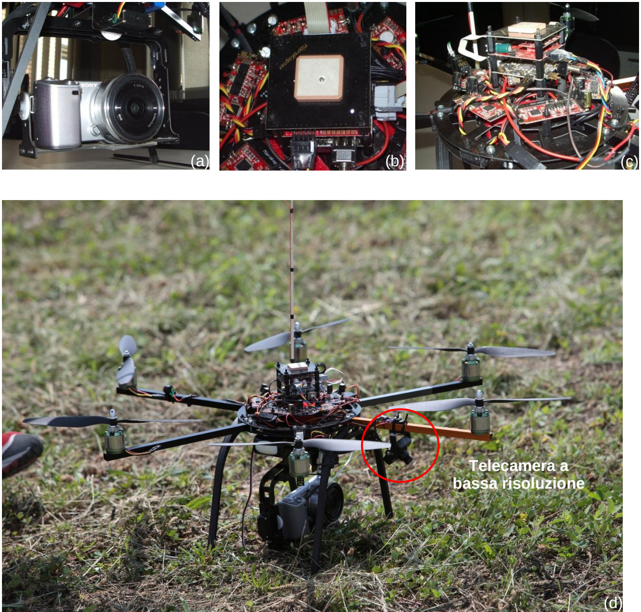
Figura 2: La camera digitale Sony NEX-5 (a), l'antenna del ricevitore GPS Ublox (b), l'elettronica di controllo (c) dal basso verso l'alto: BL, FC, NC, MK3Mag, MKGPS e l'Hexakopter di Mikrokopter (d).
