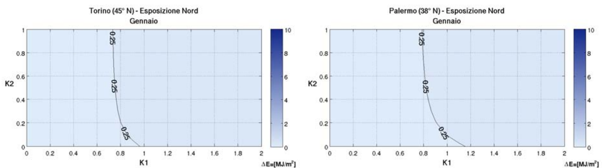
Figura 13.40 – Riduzione dell'irraggiamento medio giornaliero per una finestra quadrata con esposizione N ombreggiata da un oggetto orizzontale, nel mese di gennaio, a Torino (45° N) e a Palermo (38° N).
